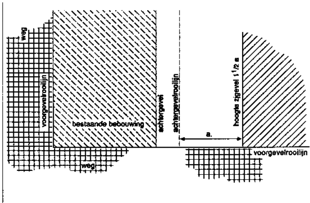
Figuur 19 Hoogte van een zijgevel tegenover een achtergevelrooilijn (artikelen 2.5.22) Toelichting
